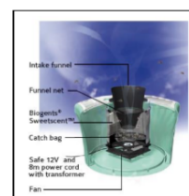
BG-MOSQUITAIRE avec un raccord électrique
